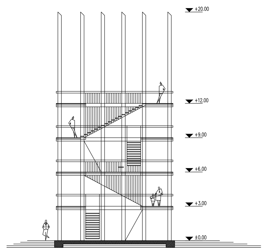
B-B metszet
