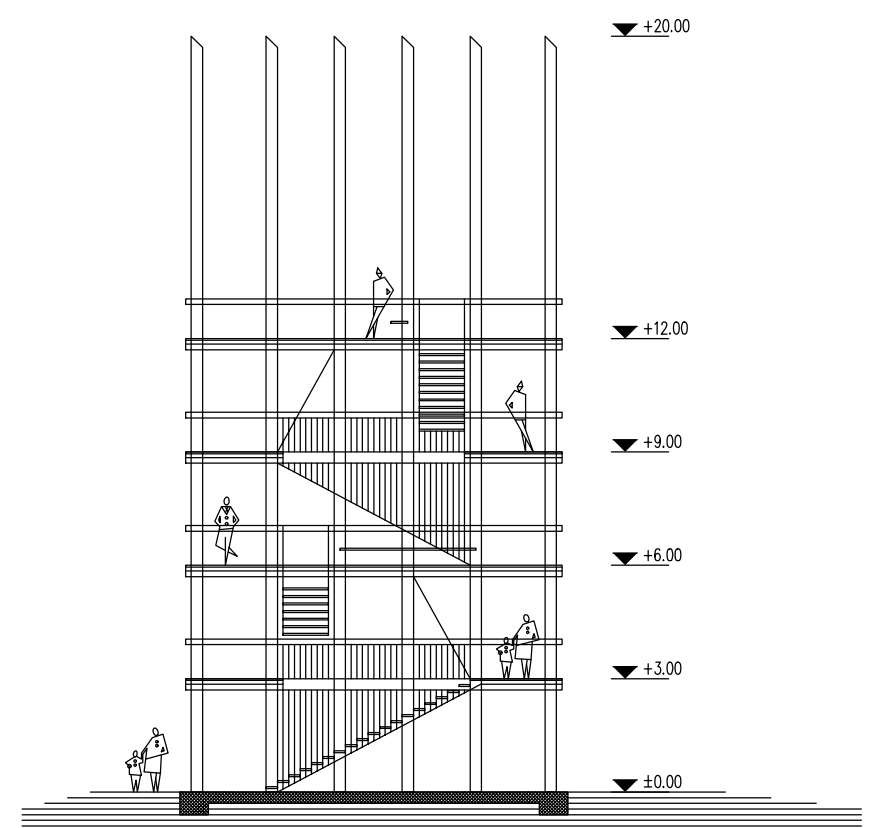
A-A metszet
