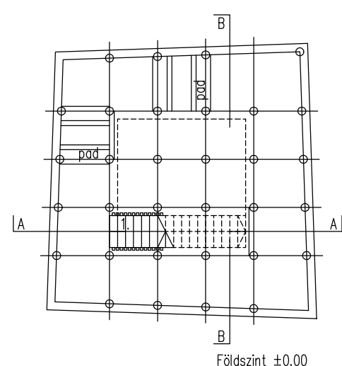
Földszint ±0.00
